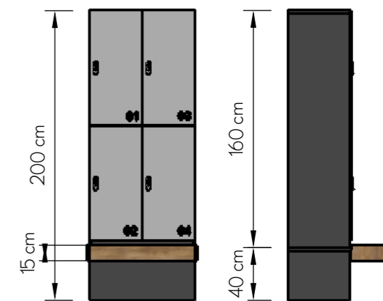
SZAFKA NA ŁAWCE LPP Z PŁYTY HPL
