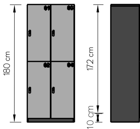
SZAFKA NA COKOLE
